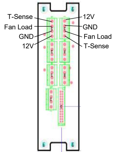
PCB Fan Connector
